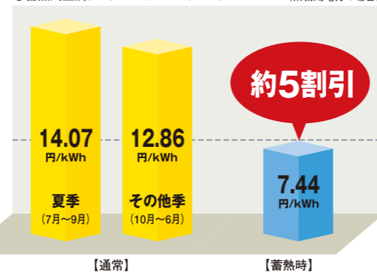
●蓄熱式空調システムのランニングコスト (業務用電力の場合)
